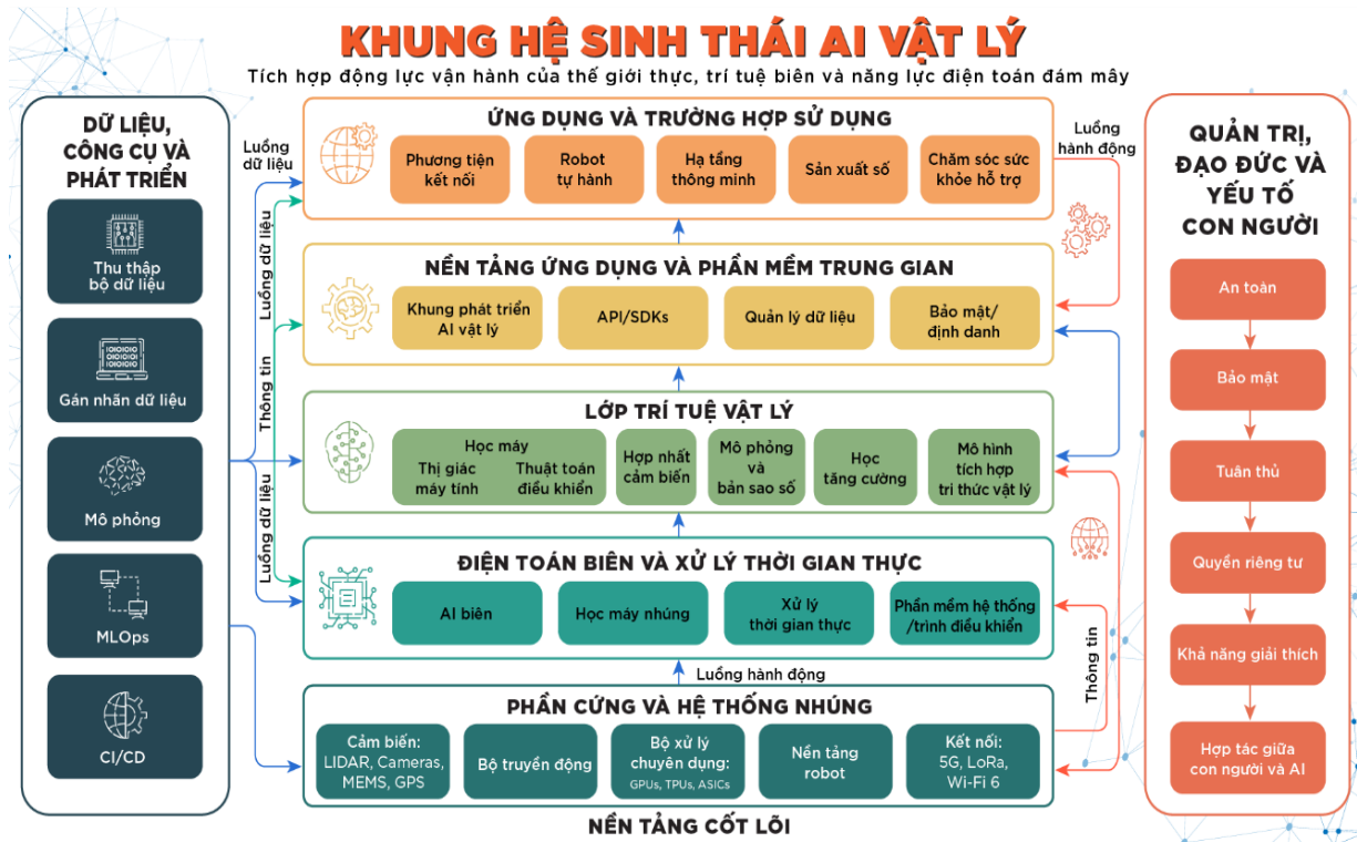
Hình 3. Hệ sinh thái của AI vật lý
