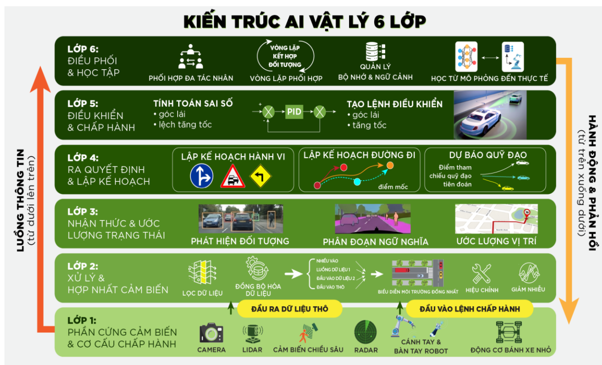
Hình 4. Cấu trúc AI vật lý 6 lớp
