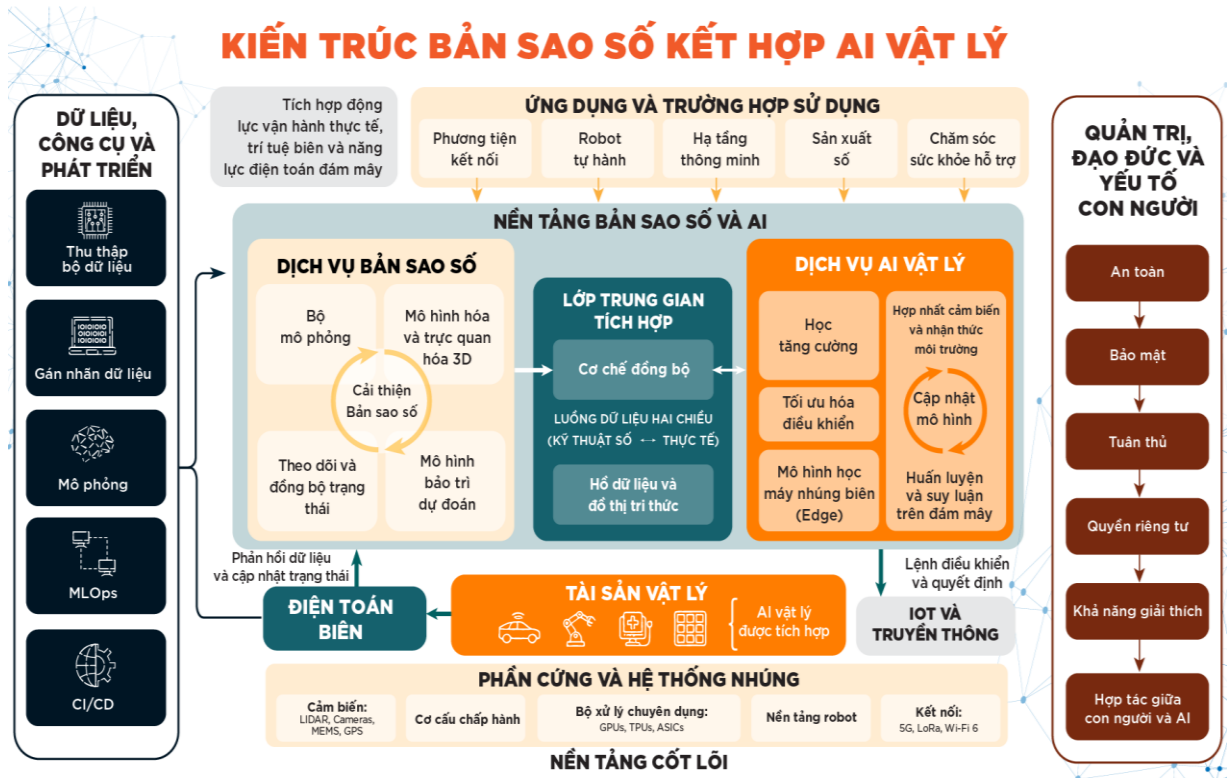
Hình 6. Sự kết hợp về mặt cấu trúc của bản sao số và AI vật lý
