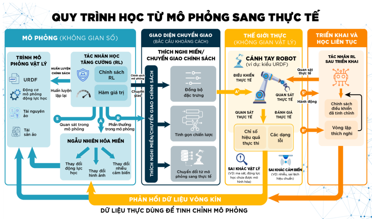
Hình 5. Cấu trúc học từ mô phỏng đến thực tế
